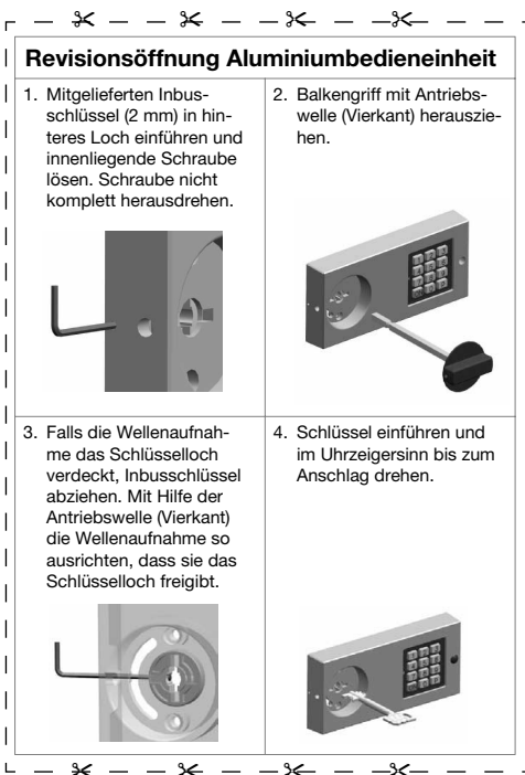
Abb. 7: Aluminiumbedieneinheit
