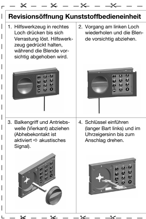
Abb. 6: Kunststoffbedieneinheit
